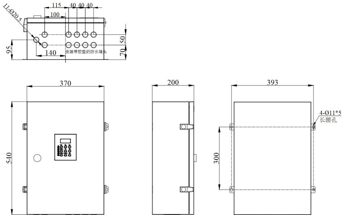
图 2.1 外形尺寸图
