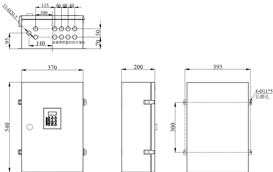
图 2.1 外形尺寸图
