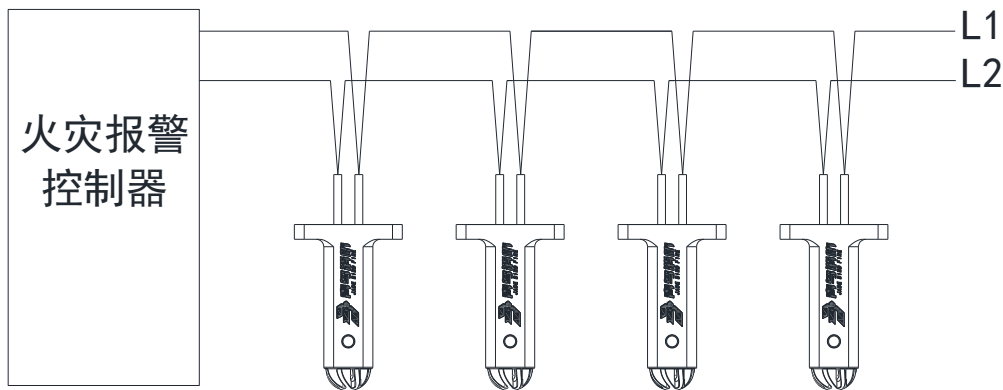
图 2 接线图例
